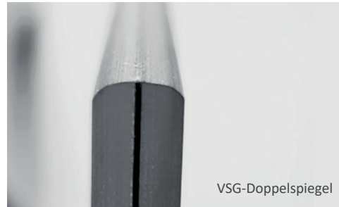
VSG-Doppelspiegel
